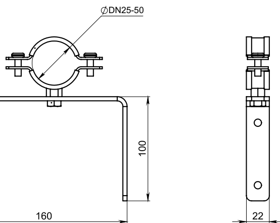
Типовой универсальный кронштейн WESER К. С трехмерным позиционированием коллектора «WPRO».
